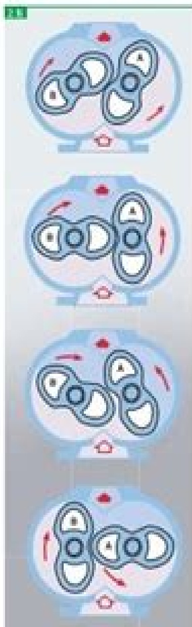
Principio de funcionamiento soplante Roots.
