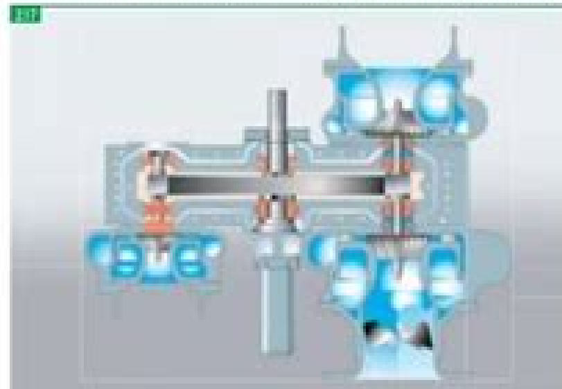
Compresor centrífugo de dos ejes.
