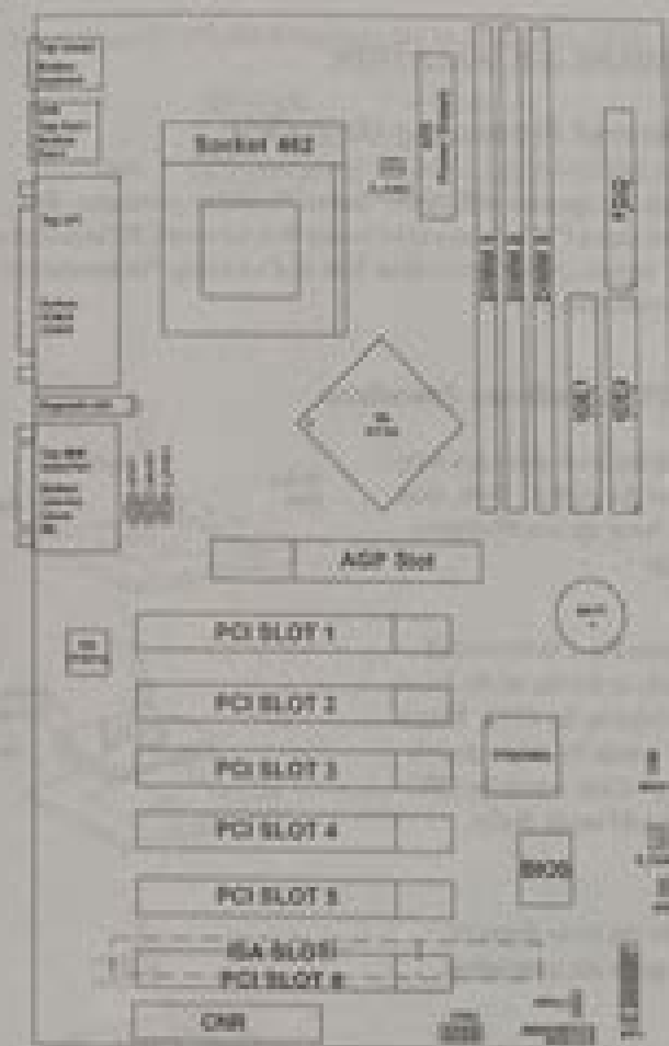
K7T PRO(MS-6330) ATX VA Mainboard
