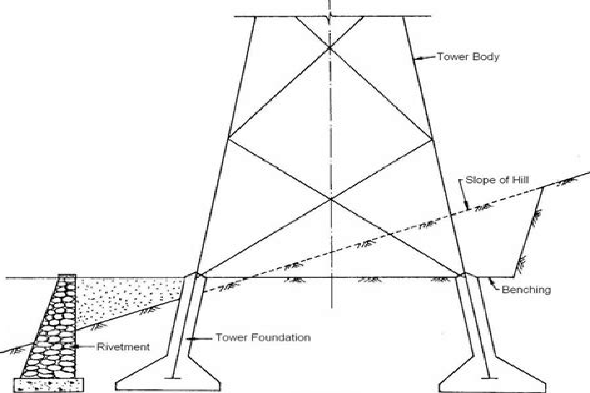
ELEVATION
