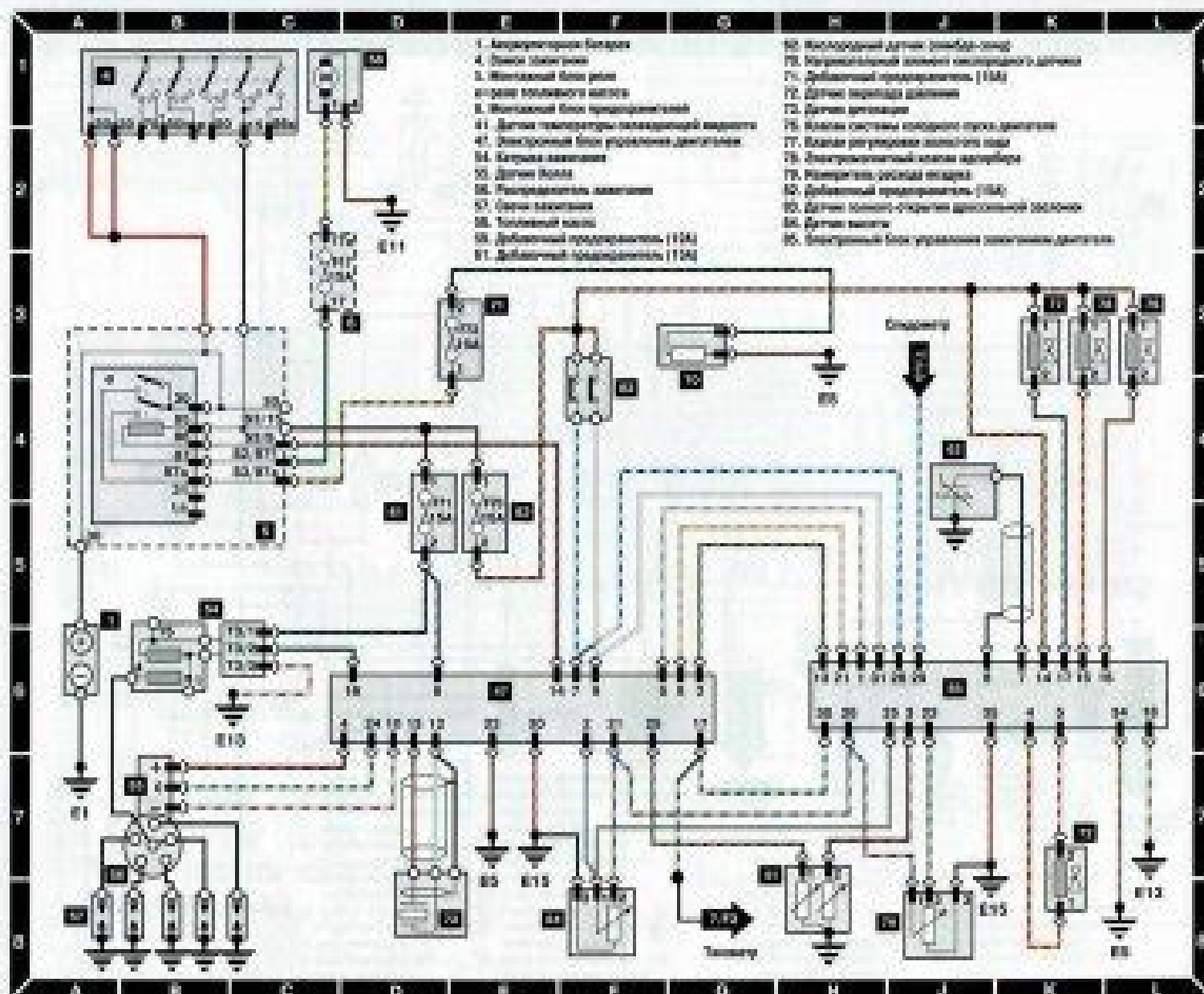
Схема 10. Система управления двигателем Audi 100 C5
